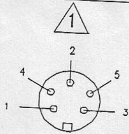
VISTA LADO SOLDADURAS CONECTOR-A
